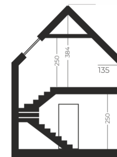
PRZĘKRÓJ
